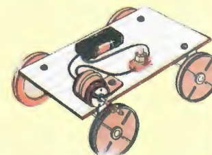
COCHE JUGUETE Coche de muy fácil construcción que derrapa sobre una rueda
